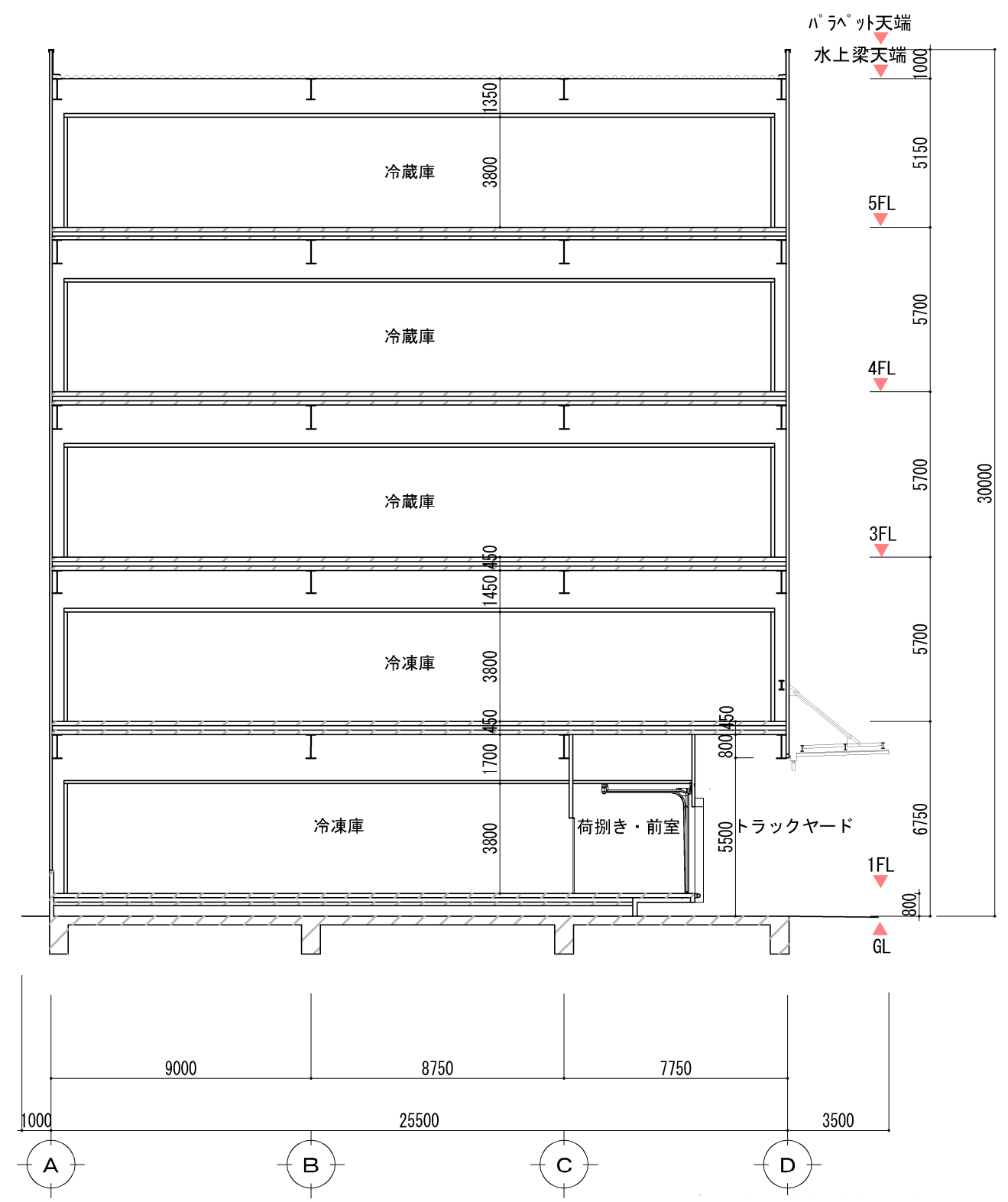
A-A' 断面図
