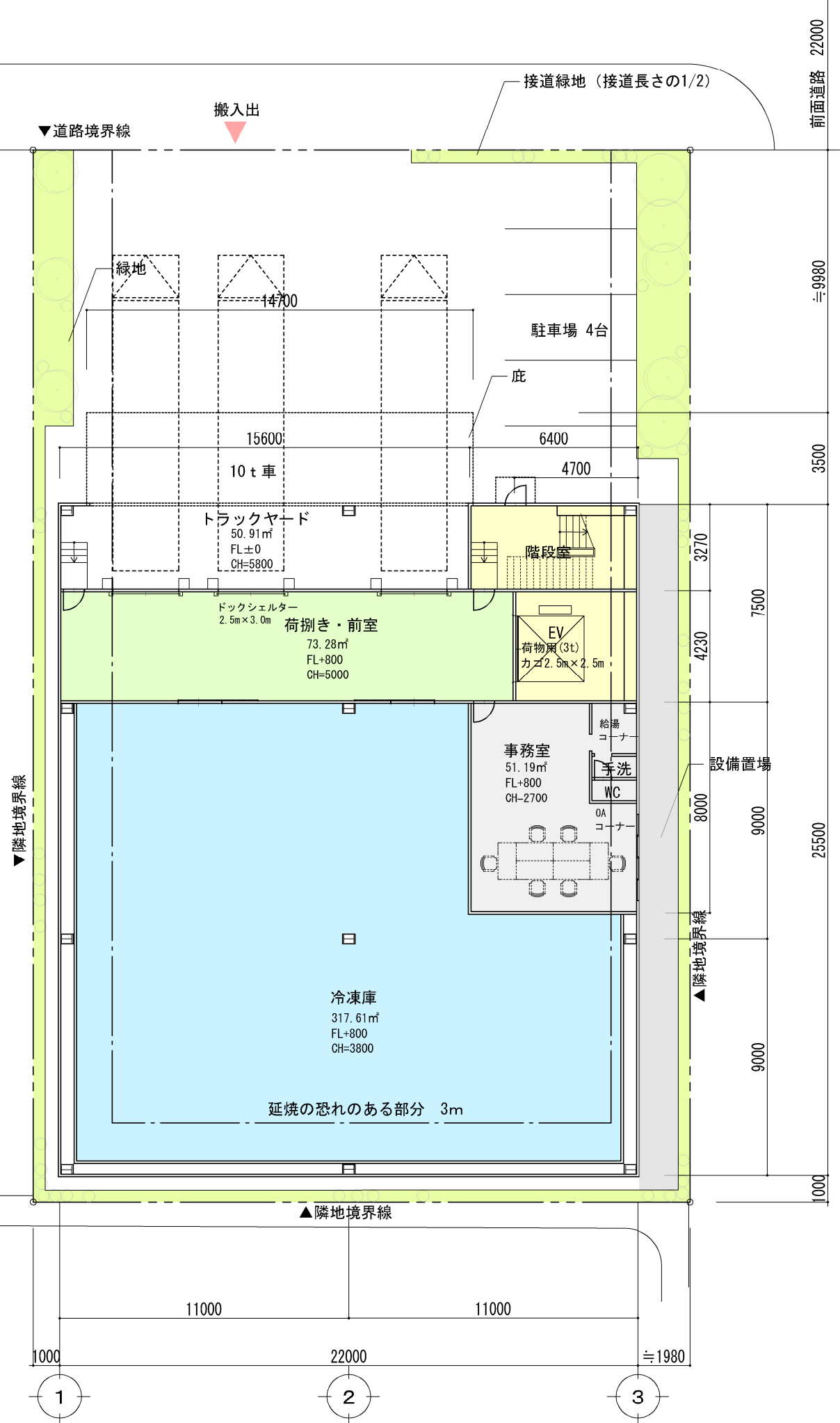
1階平面図
