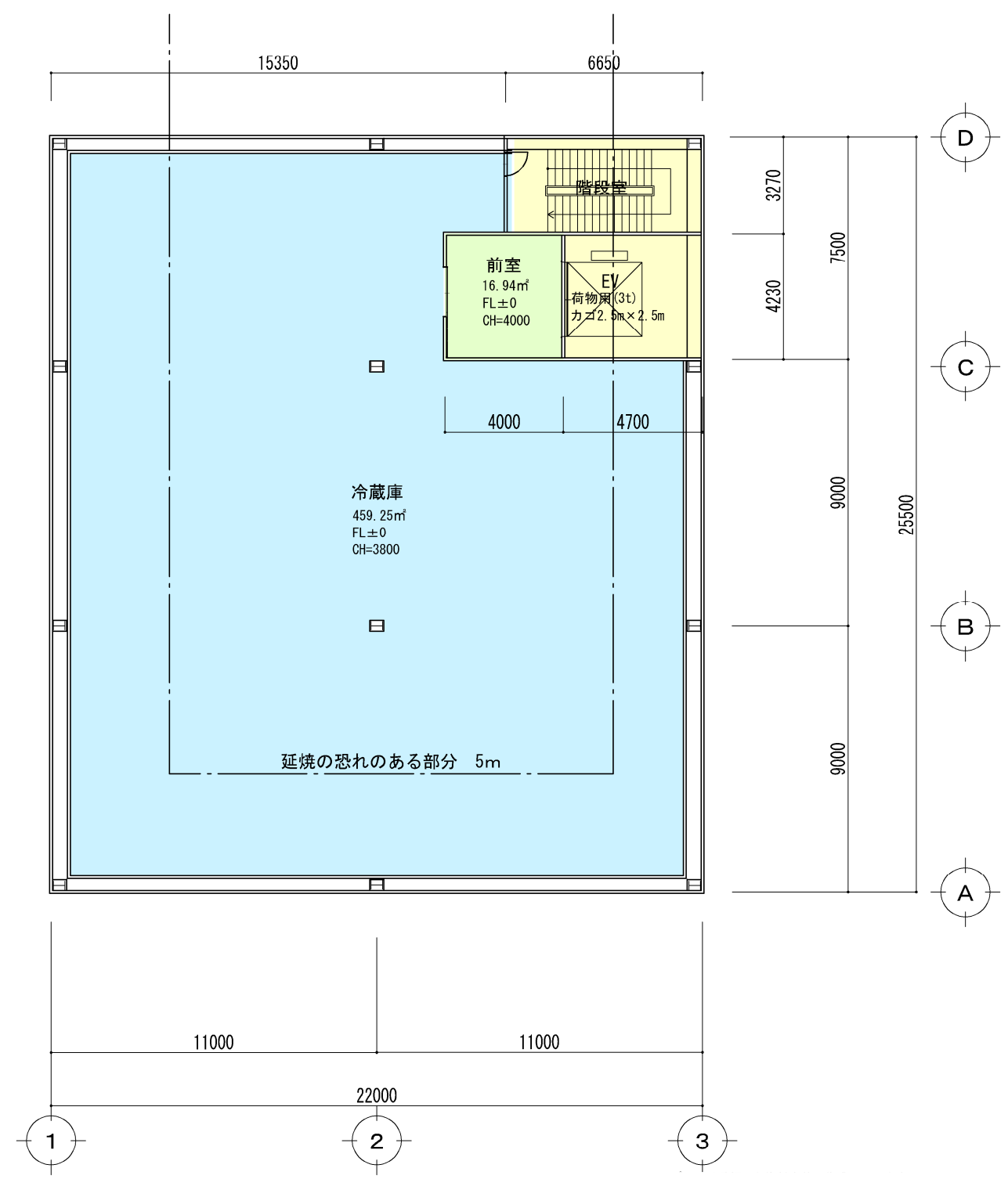
3~5階平面図
