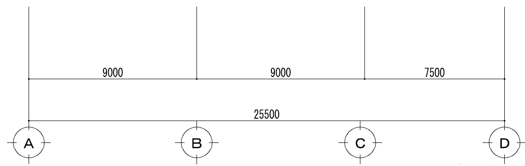
東面 立面图
