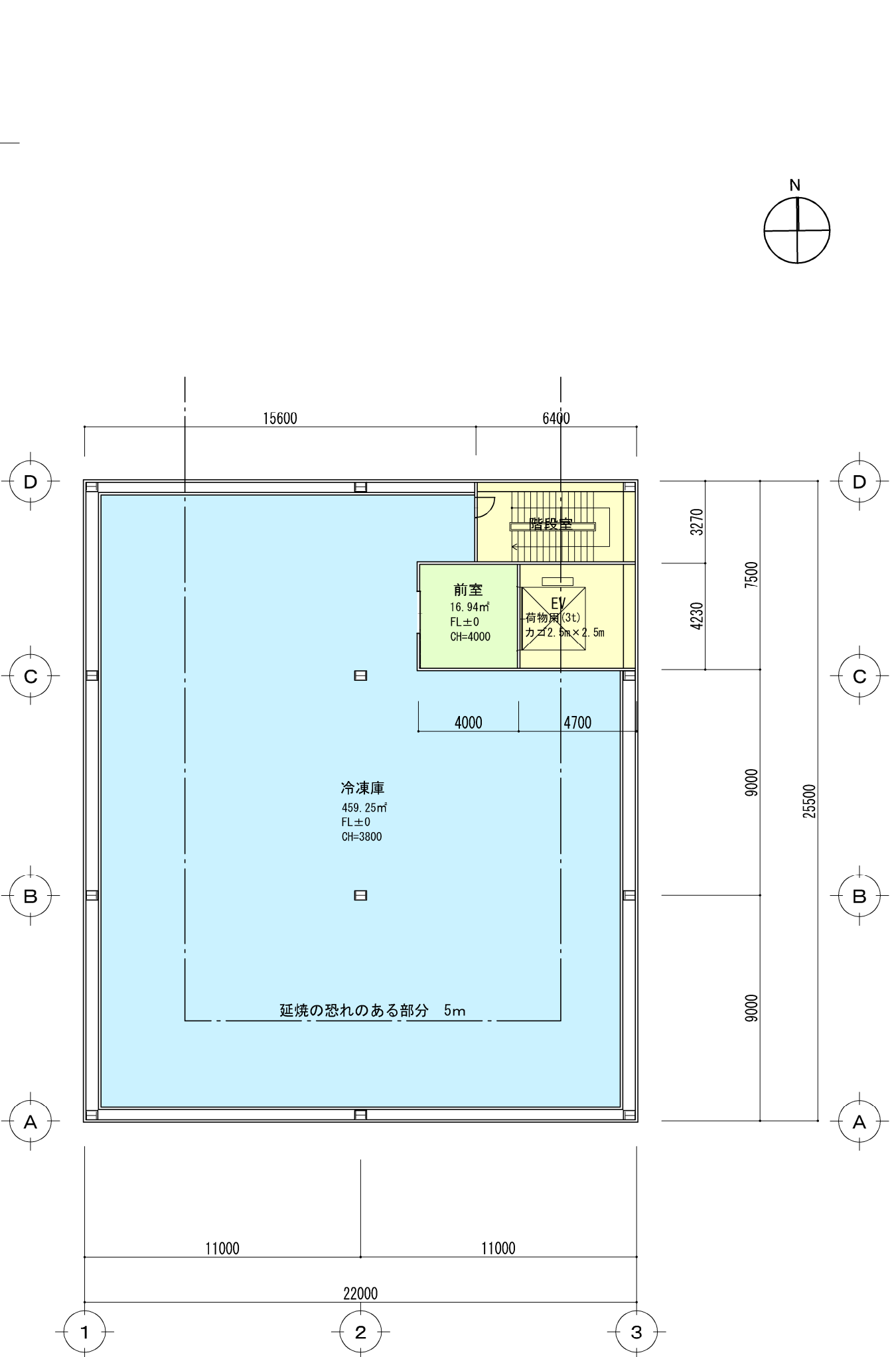
2階平面図
